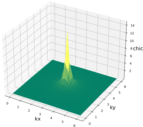
Fig. 4.1: \chi_c(\vec{q})
